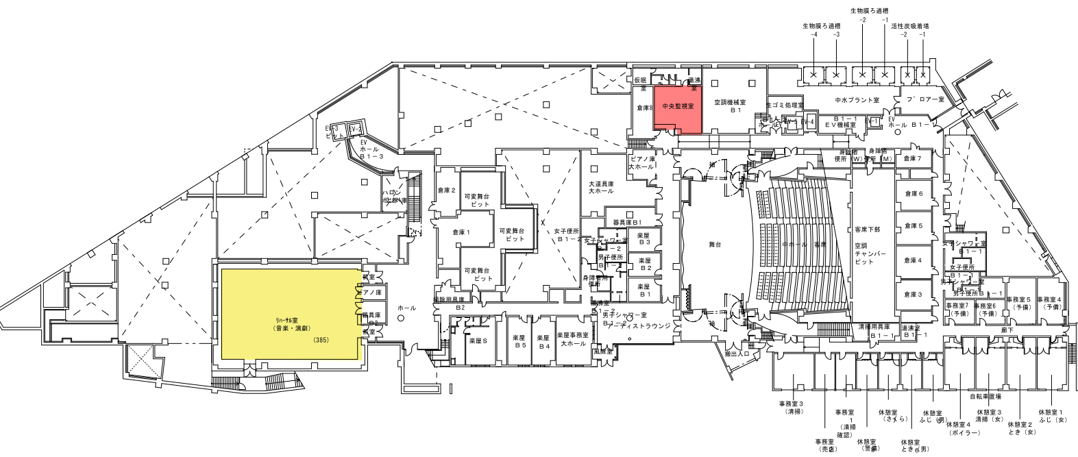
カルチャー棟 地下1階 平面図 (1:500)
