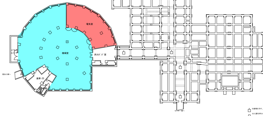
宿泊D棟・国際交流棟 地下1階平面図 (1:400)
